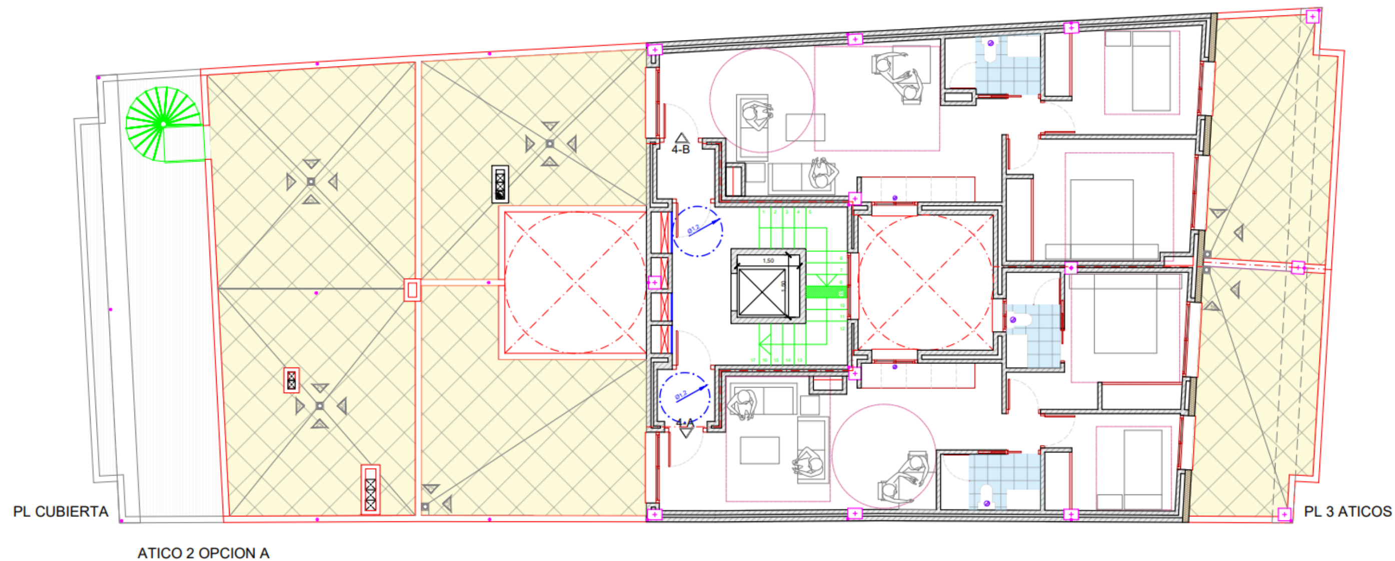
PLANTA 4ª ÁTICOS
